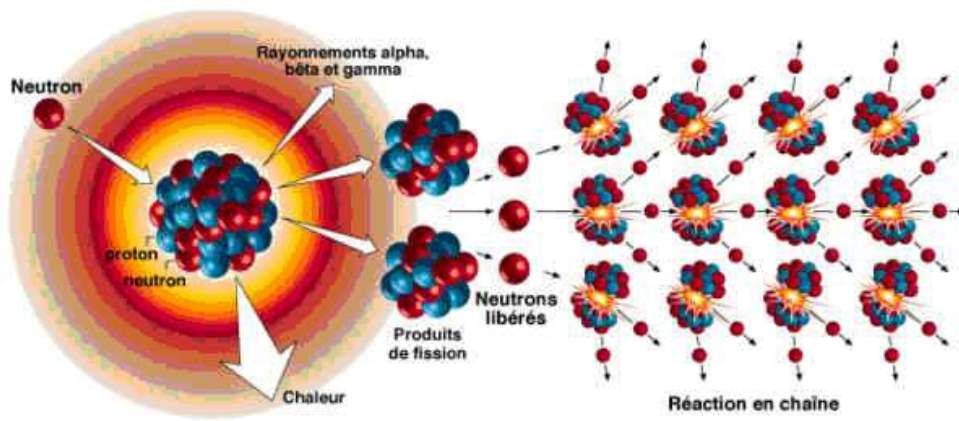
Fission
