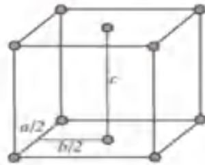
(c) Maille à base centrée, S
