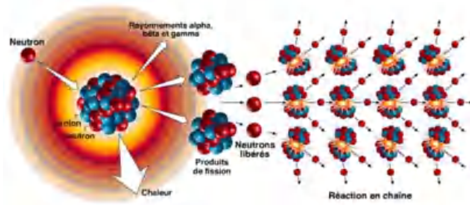
Fission
