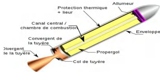
Schéma d'un propulseur a propergol solide
