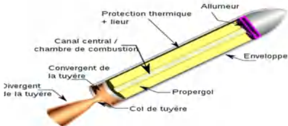
Schéma d'un propulseur a propergol solide
