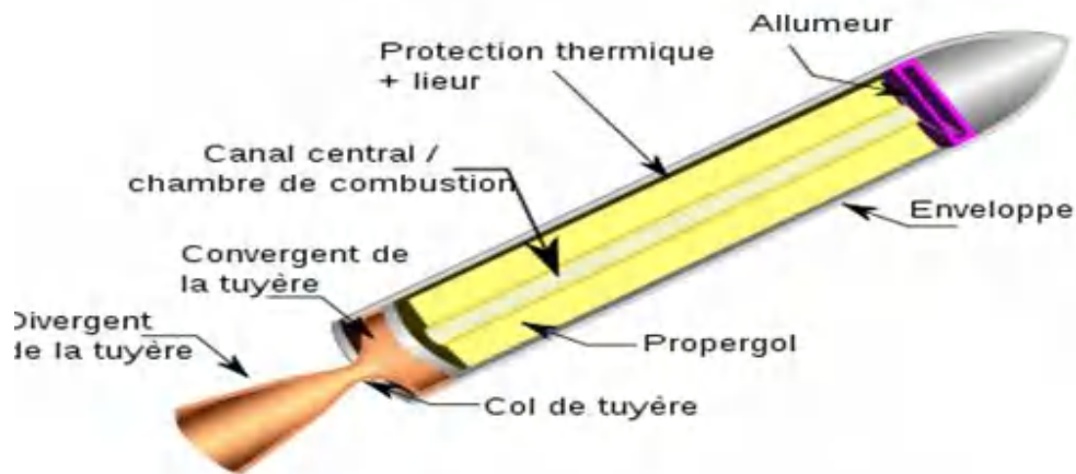
Schéma d'un propulseur a propergol solide
