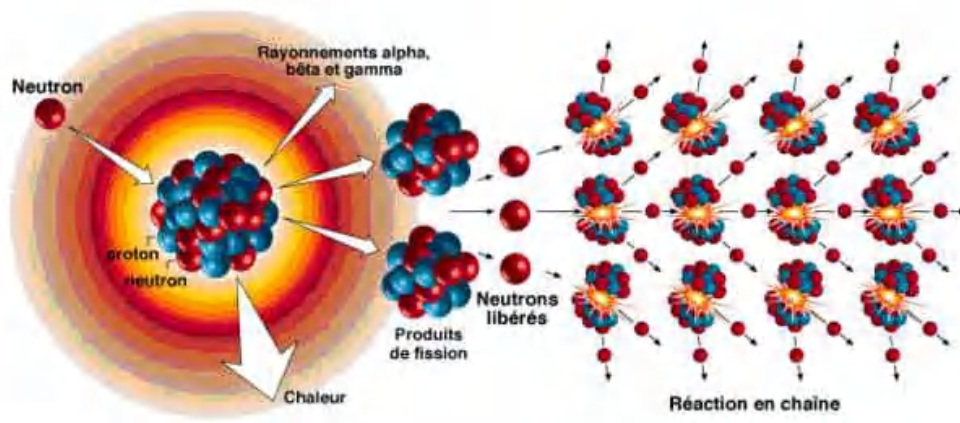
Fission
